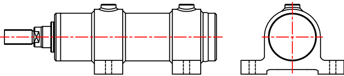
STYLE LM LUG MOUNT
